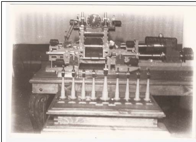
Foto: Maqueta del Tren de Laminación Blooming
